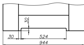
křídlo SEMPRE „90“ s ventilačním seříznutím
