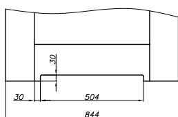
křídlo ARCO „80“ s ventilačním seříznutím
