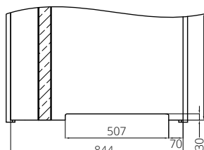
křídlo IMPULS W13 „80“ s ventilačním seříznutím
