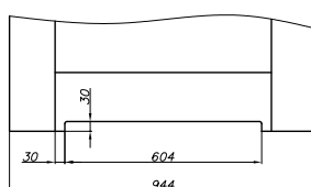
křídlo ARCO „90“ s ventilačním seříznutím
