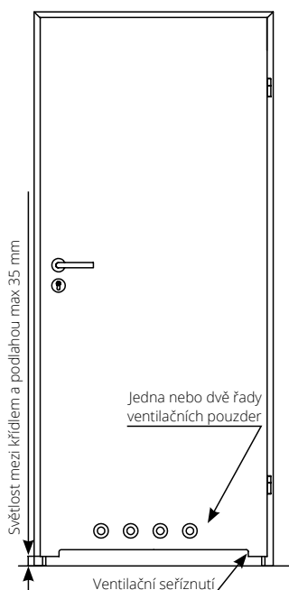
křídlo ARCO „80“ s ventilačním seříznutím
