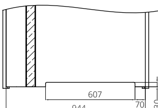
křídlo IMPULS W13 „90“ s ventilačním seříznutím
