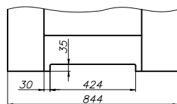
křídlo SEMPRE „80“ s ventilačním seříznutím
