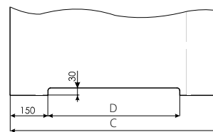
křídlo CAMBIO DUO s ventilačním seříznutím
