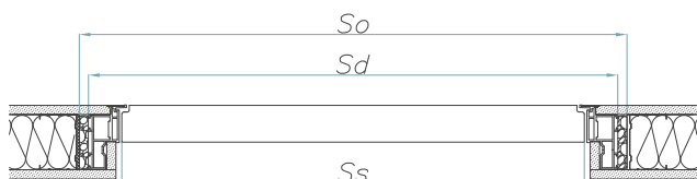
dveře ODW (otevření dovnitř)
