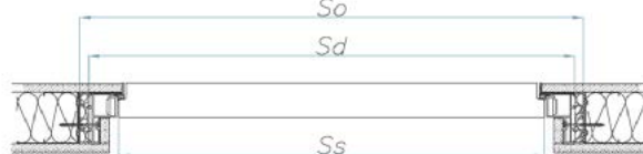
DVEŘE HARMONY INVEST PRO otvírání dovnitř s obložkovým panelem
