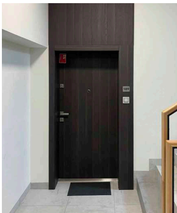
dveře RC3, verze W0, pevná dřevěná zárubeň
