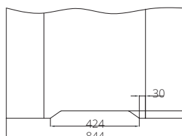
křídlo „80” s ventilačním seříznutím
