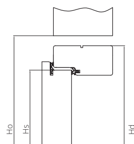
dveře SEGURO, verze VD9, pevná dřevěná zárubeň
