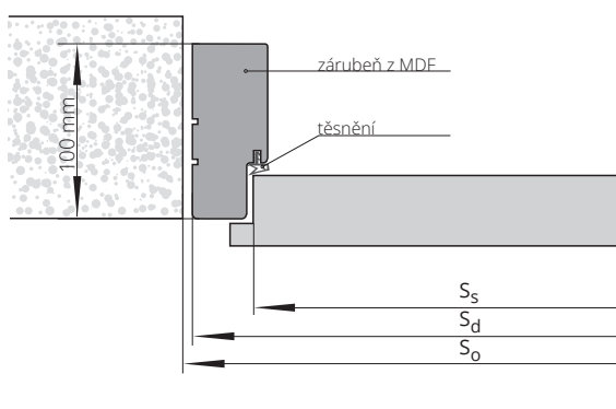
PEVNÁ MDF:
