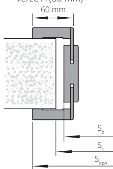
Tunel ZN s lištami verze A (60 mm)
