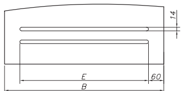
ventilační spára v bezfalcových křídlech
