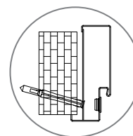
montážní otvor na kotvu ve falci zárubně
