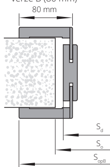
Tunel ZN s lištami verze B (80 mm)
