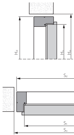
EI30 PLUS, EI60 PLUS, RC3, GAMMA, DECO INVEST, CERBER PLUS ZÁRUBEŇ KOVOVÁ PEVNÁ
