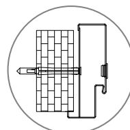
montážní otvor na kotvu ve středu profilu na celé zárubně
