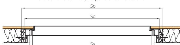
Dveře otvírávé dovnitř pro panelovou konstrukci
