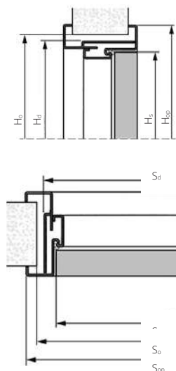
EI30 PLUS, EI60 PLUS ZÁRUBEŇ KOVOVÁ NASTAVITELNÁ
