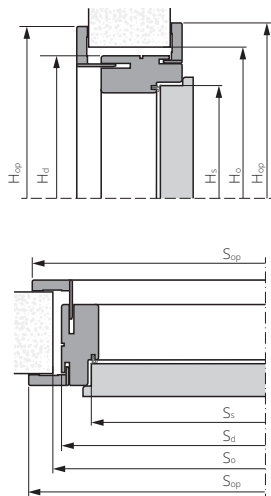
ZVUKOTĚSNÉ TYP A, B ZÁRUBEŇ DIN ZP NASTAVITELNÁ
