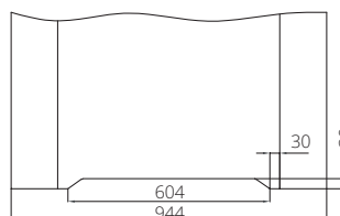
křídlo „90” s ventilačním seříznutím
