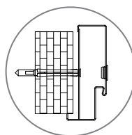
montážní otvor na kotvu ve středu profilu na čele zárubně
