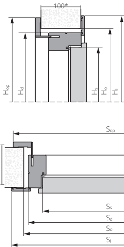
FR EI30, EI 30 PLUS, EI 60 PLUS, B-30, C-30, RC3, SR 37 dB, SR 42 dB, CERBER PLUS, GAMMA ZÁRUBEŇ DŘEVĚNÁ
