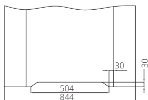
křídlo „80” s ventilačním seříznutím
