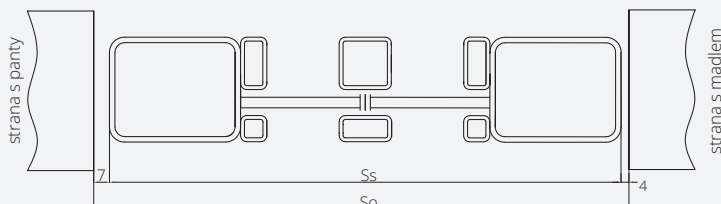
DVEŘE ZAVŘENÉ
