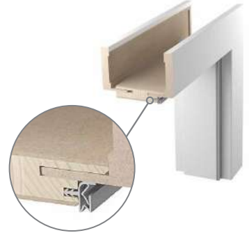
SOLID DIN DUO vyrobena z vysoce kvalitního vrstveného dřeva (základní část), lišty vyrobeny z vysoce kvalitní MDF
