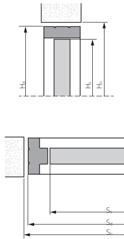
DVEŘE KYVNÉ ZÁRUBEŇ DŘEVĚNÁ PEVNÁ
