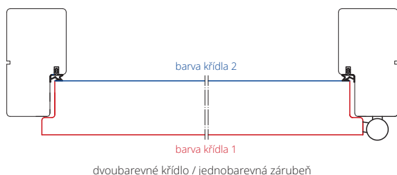
dvoubarevné křídlo, jednobarevná zárubeň
