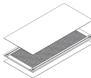
KONSTRUKCE KŘÍDLA
