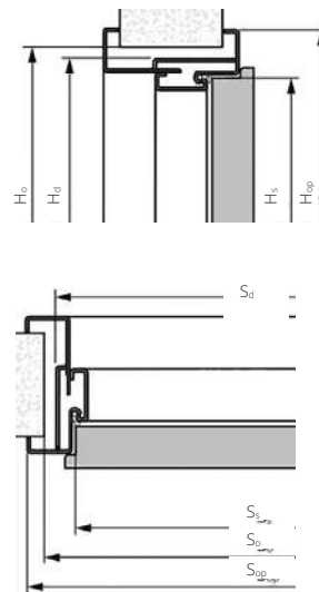
DVEŘE KYVNÉ ZÁRUBEŇ DŘEVĚNÁ PEVNÁ
