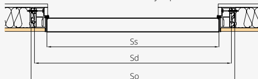
DVEŘE HARMONY INVEST PRO otvírání ven s obložkovým panelem
